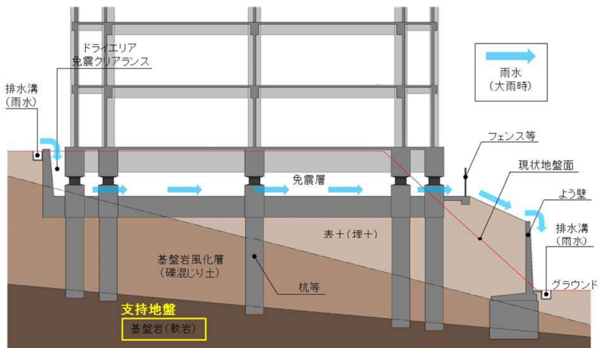
図 6 断面モデル
