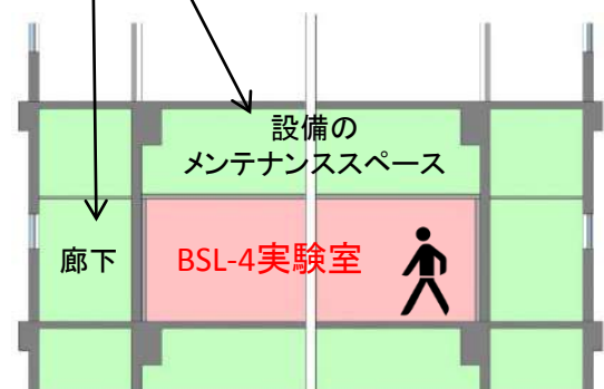
BSL-4施設の断面図
